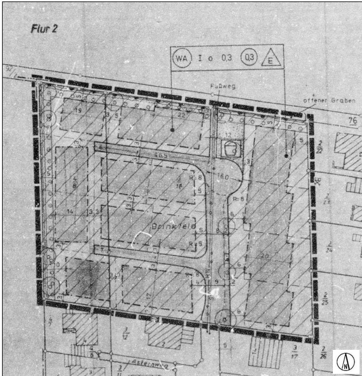
Abb.: Auszug aus dem rechtsverbindlichen Bebauungsplan Nr. H3A „Beckfeld II“
